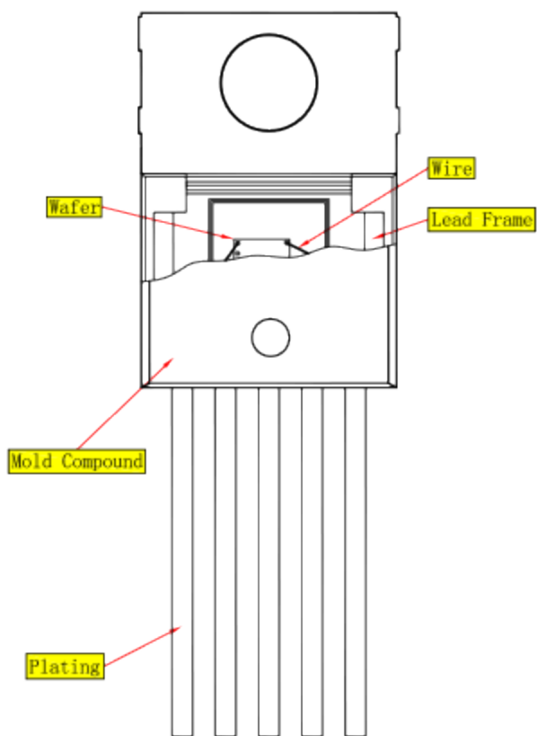
正视图
