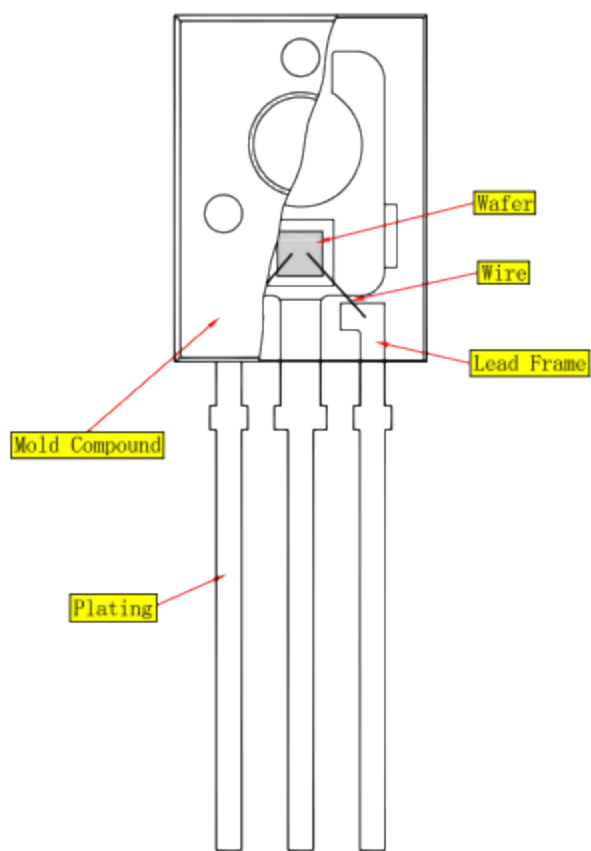
正视图
