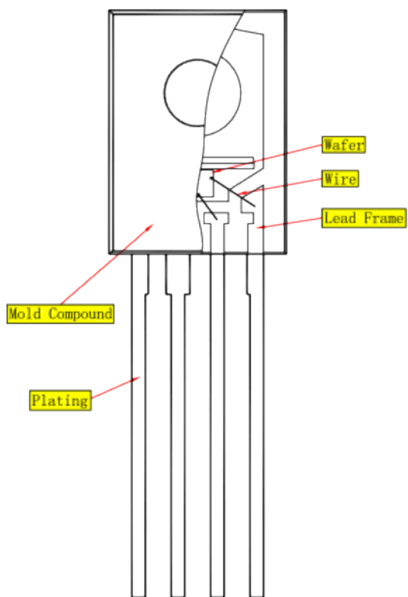
背视图
